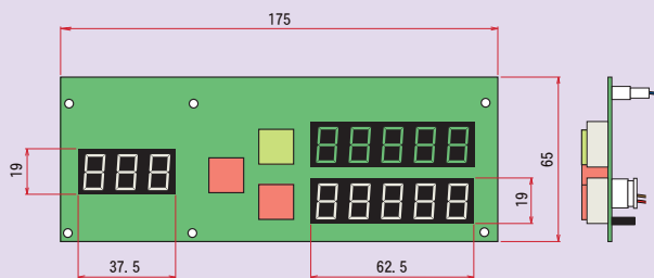
* デジタル料金 2 段表示基板 (MH-15A)
