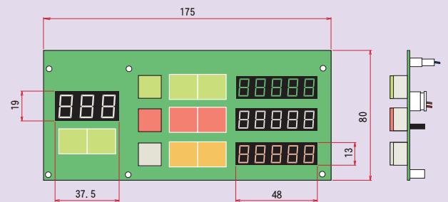
* デジタル料金 3 段表示基板 (MH-15B)
